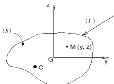
Figure 8 : section générale.
