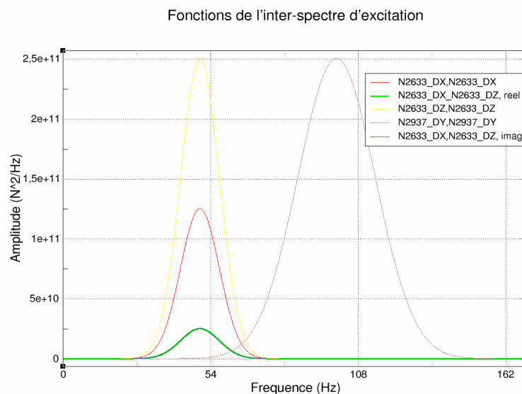
Figure 5.2.1-a : inter-spectre d'excitation.
