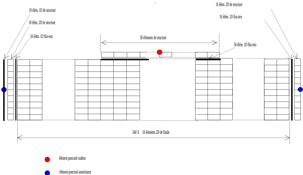
Figure 3.2-a : Maillage bidimensionnel du modèle d'oscillateur fluidélastique
