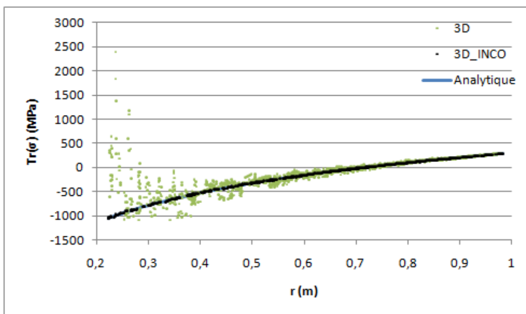
Figure 4.4-a : Trace des contraintes en Mpa pour les formulations 3D, 3D_INCO et la solution analytique
