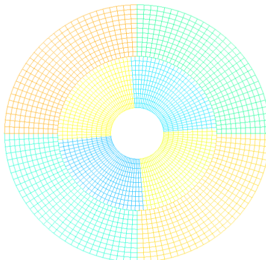
Figure 6.2-a: Le maillage de la modélisation D
