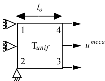
Figure 1.3-1: Conditions limites et chargement
