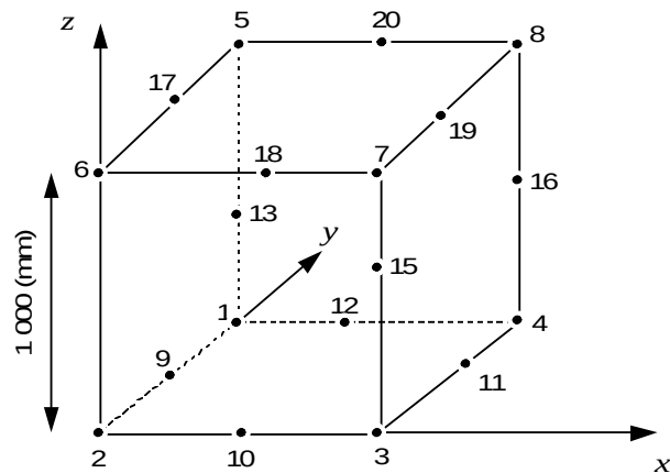
Figure 3.1-1: Maillage de la modélisation A
