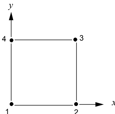
Figure 4.1-1: Maillage de la modélisation B
