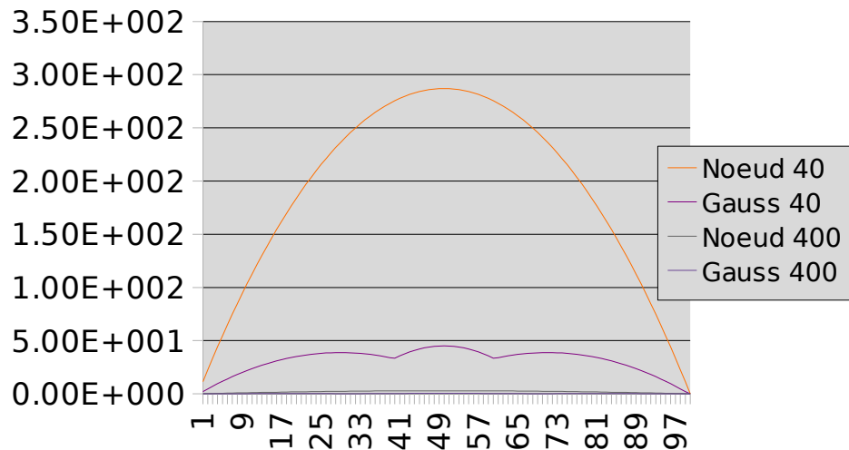
Figure 5.4-2: Evolution de la pression de contact lors de la rotation pour 160 et 1600 éléments sur la circonférence R=R_2 . Avec le maillage à 160 éléments on atteint une erreur de 30000 % avec intégration aux noeuds et 5000% avec intégration à 2 points de Gauss pour une erreur inférieure à 4% sans rotation avec compatibilité des maillages des surfaces maître et esclave.
