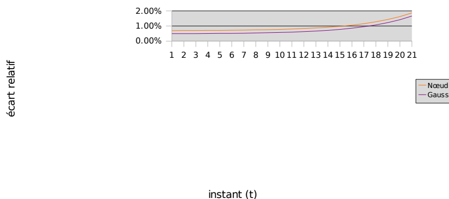
Figure 3.4-1: évolution de l'écart entre la solution analytique et la solution donnée par Code_Aster pour une intégration aux nœuds et aux points de Gauss.
