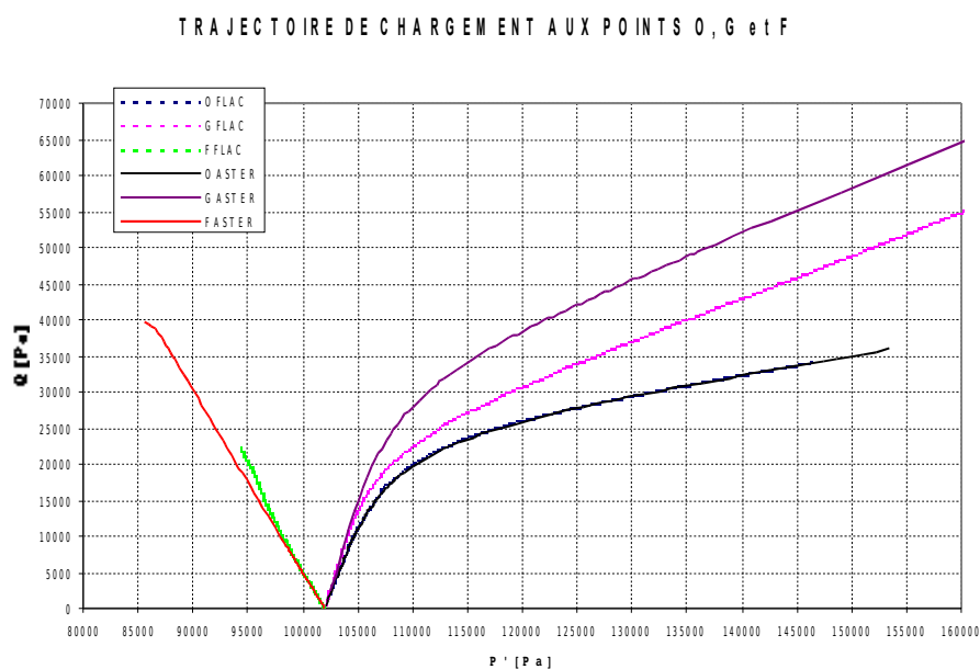
Figure 3 : comparaison des trajets de chargement dans le plan (P', Q) aux points O , G et F donnés par Code_Aster et FLAC pour la modélisation A.
