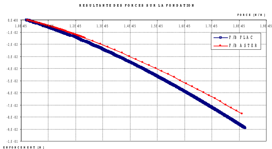
Figure 4 : comparaison des résultantes des forces exercées sur la fondation données par Code_Aster et FLAC pour la modélisation A.
