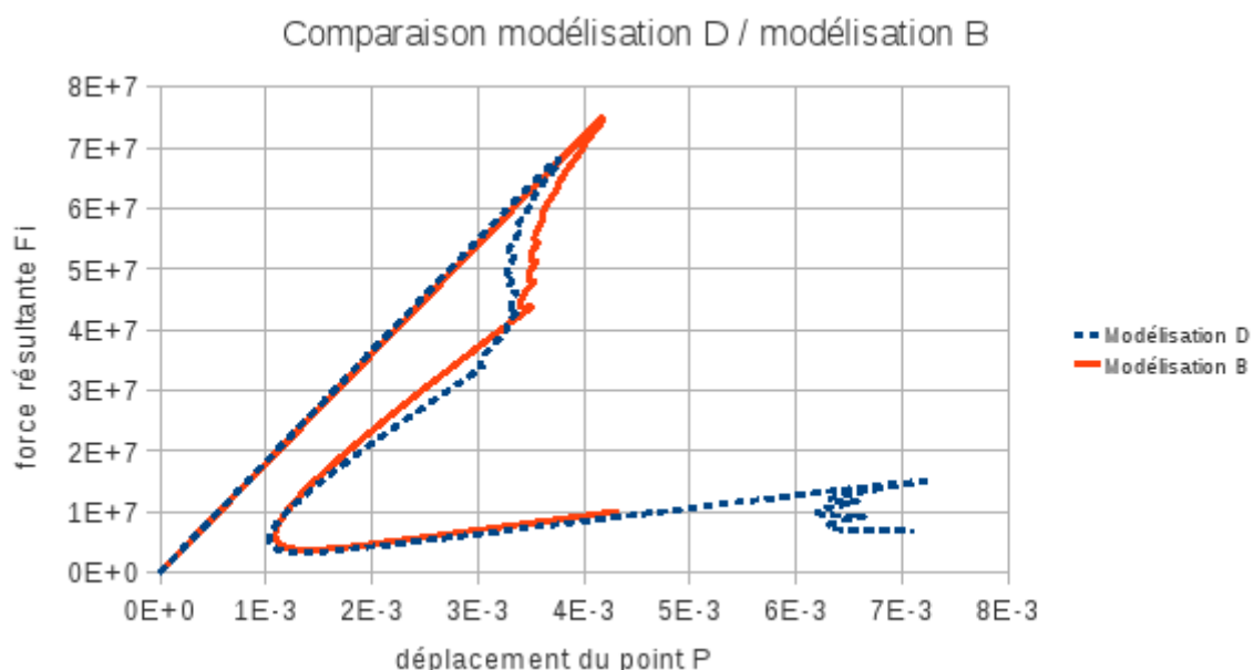
Figure 6.3-a: comparaison éléments de joint avec éléments à discontinuité interne.
