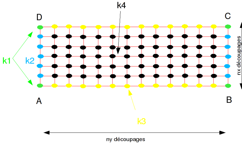
Figure 2.2-b : Discrétisation de la plaque dans le plan (x, y) .
