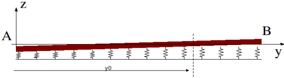
Figure 2.2-a : Schéma de la plaque et des ressorts après chargement.
