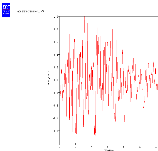
Figure 1.3-a : Accélérogramme LBNS
