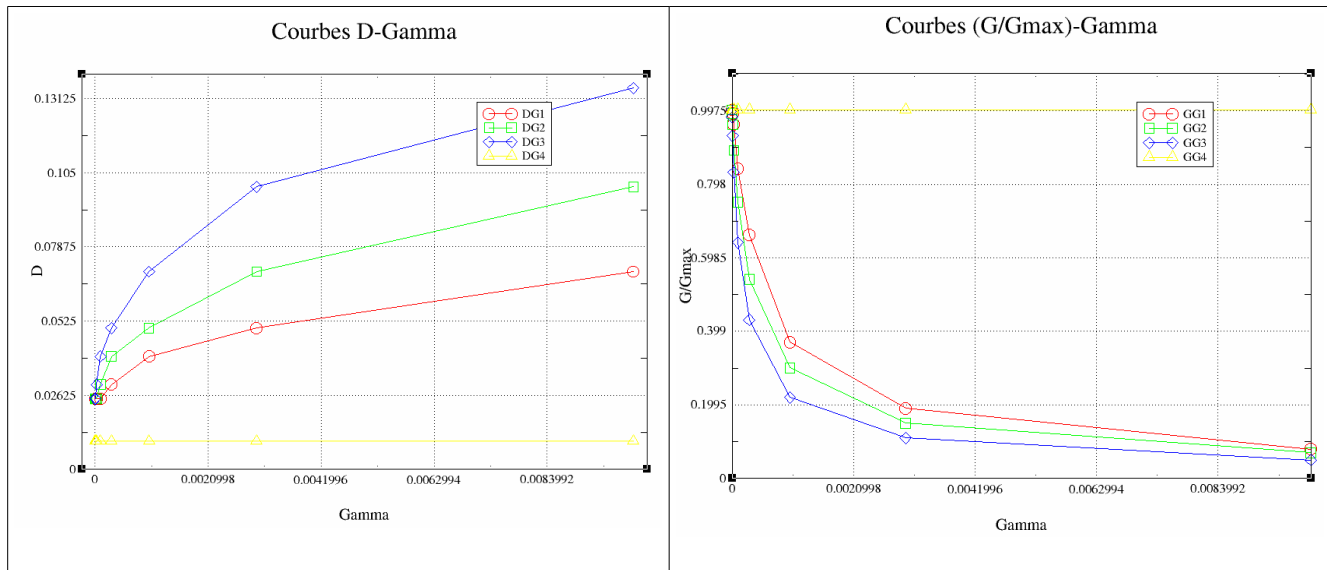
Caractéristiques D-Gamma et (G/Gmax)-Gamma par matériau constitutif des couches
