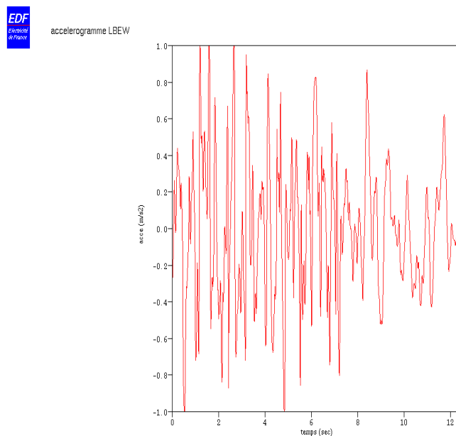
Figure 1.3-b : Accélérogramme LBEW
