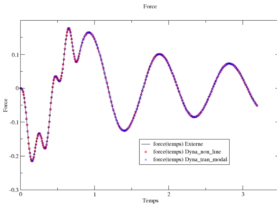
Figure : Réponses (force en fonction du temps), calculées par une méthode externe et par avec les commandes et DYNVIBRA.
