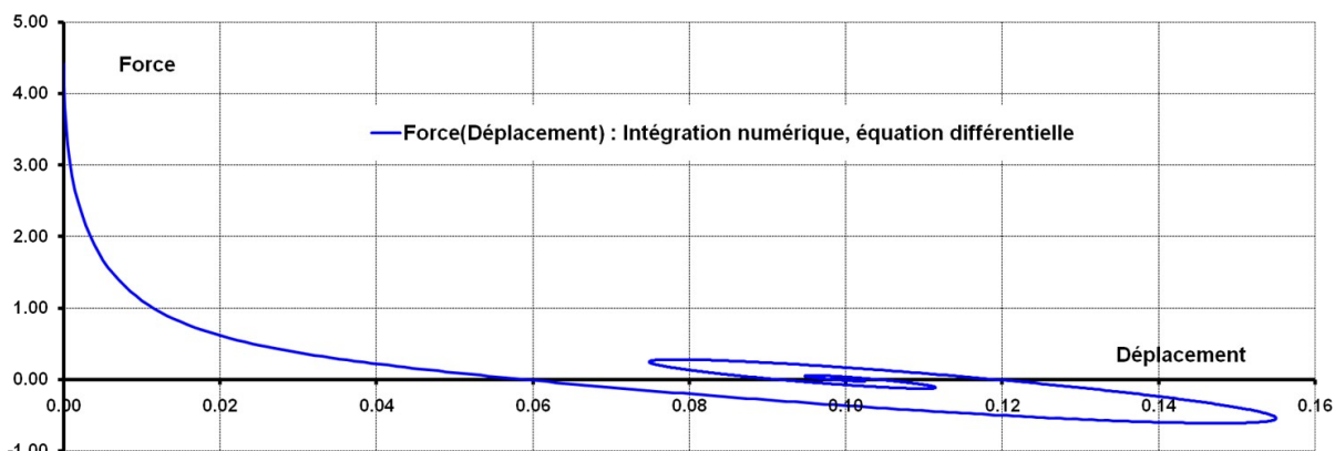
Figure 2.1.1-b : Évolution de l'effort en fonction du déplacement
