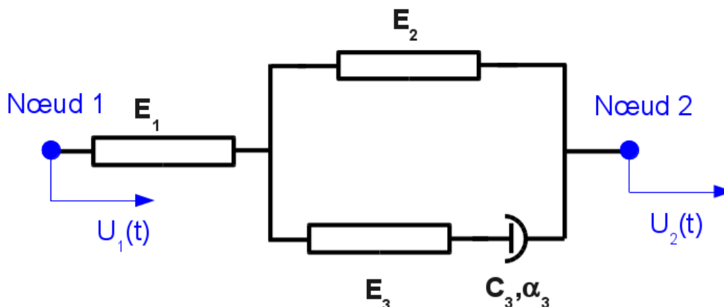
Figure Modèle rhéologique de l'amortisseur visqueux.
