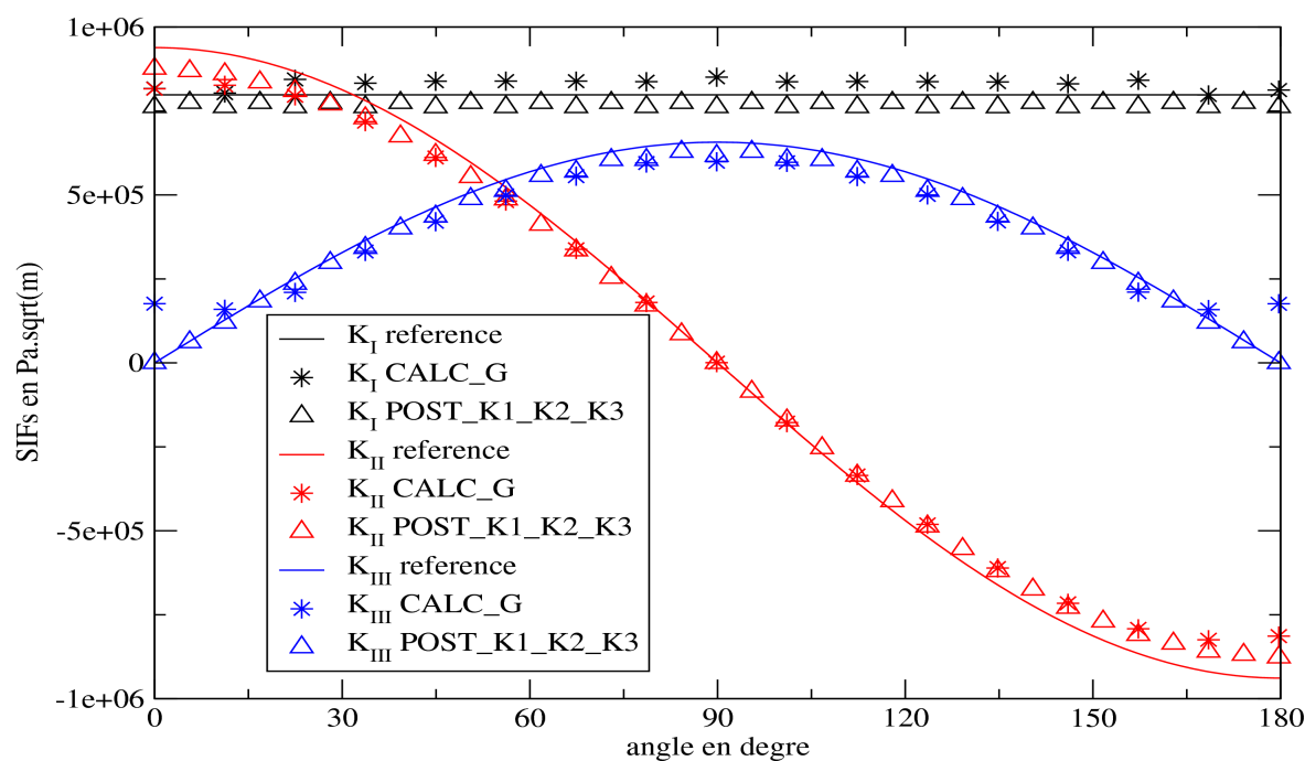
Figure 3.4-5: SIFs le long du fond de fissure (FEM)
