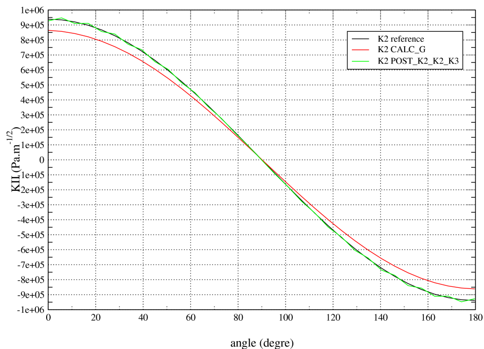
Figure 3.4-3: K2 le long du fond de fissure
