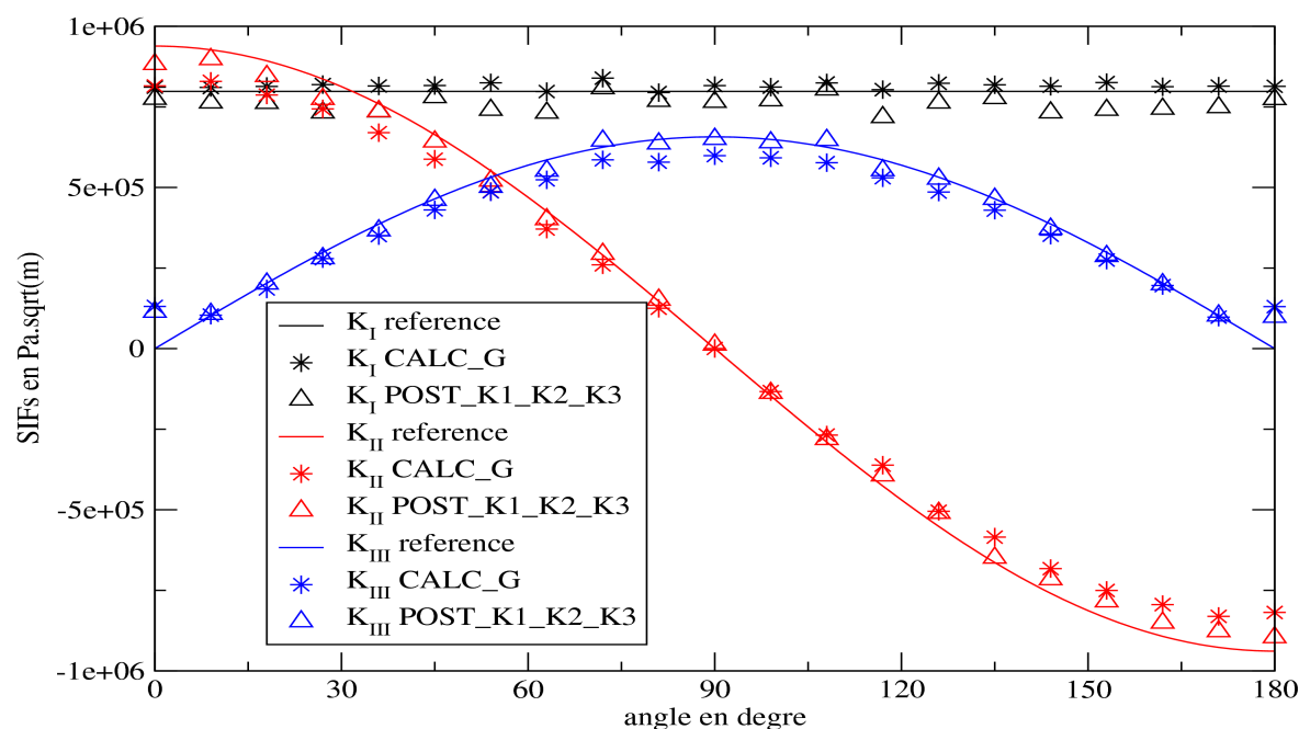
Figure 4.4-1: SIFs le long du fond de fissure (FEM)
