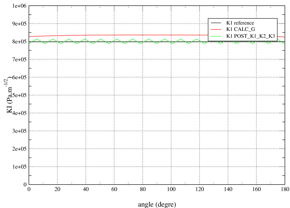
Figure 3.4-2: K1 le long du fond de fissure
