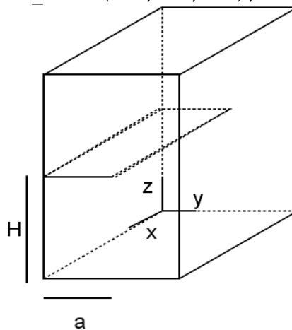
Figure 3.2-a : Barreau fissuré
