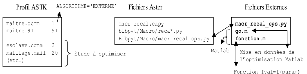
Figure 7.2.1-a: MACR_RECAL « Algorithme externe »
