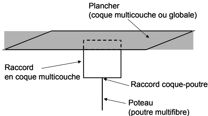
Figure 3.6.2-a : liaison poteau – plancher.
