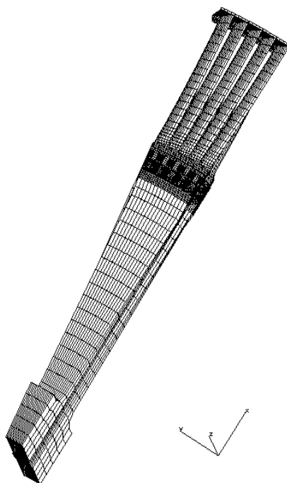
Figure 5.1-1: Maillage d'un paquet d'aillette de l'aubage 5-12
