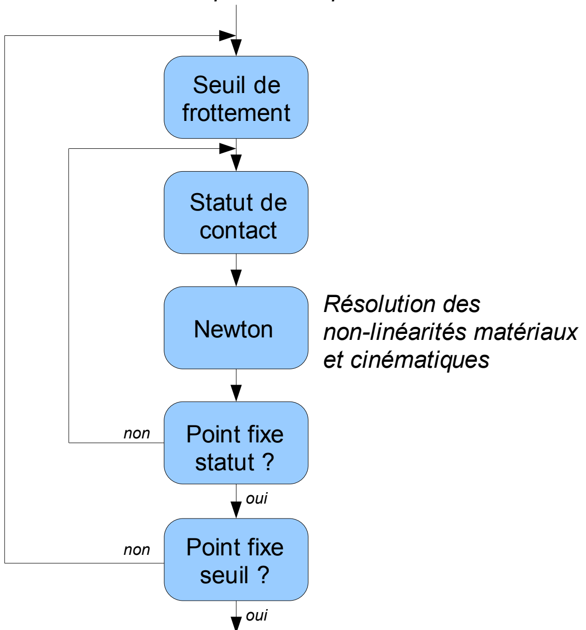
Figure 3.1.3-1: Algorithme général d'un pas de temps en formulation continue avec point fixe (petits glissements)
