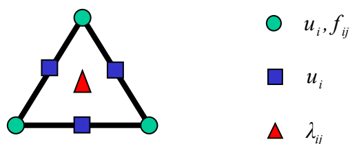
Figure 1.3-a : Discrétisation élément fini du modèle second gradient pour les déformations planes
