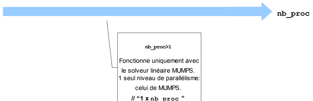
Figure 4-3b. INFO_MODE seul ou en pré-traitement de CALC_MODES avec option ' BANDE ' découpée en sous-bandes.
