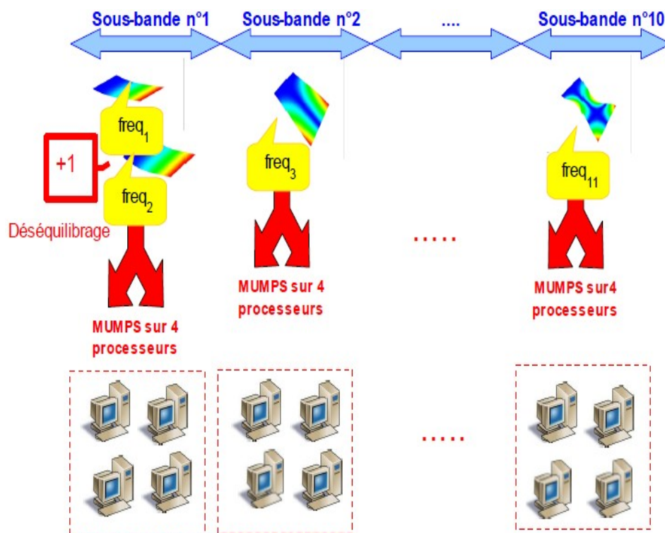
Figure 4-9. Déséquilibre de charge « fréquences/sous-bandes ».
