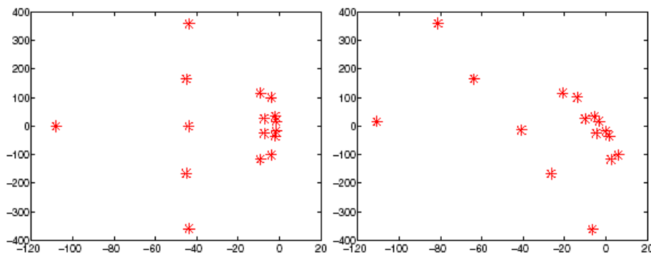
Figure 2.2-1. Exemples du spectre d'un QEP ( n=8 ) d'une modèle simplifié d'enceinte nucléaire[TM01]. Figure de gauche, on est dans le cas n°3 du tableau 2.2-1. Celle de droite, on rajoute à \mathbf{K} de l'amortissement hystérétique donc apparaissent des modes dépareillés (cas général n°1).
