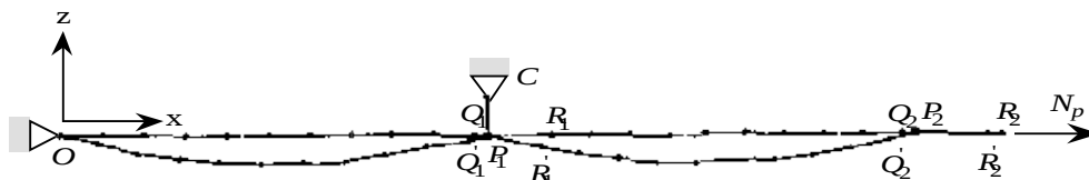
Figure 7-a : Equilibre d'un câble à deux portées, soumis à une tension de réglage donnée.
