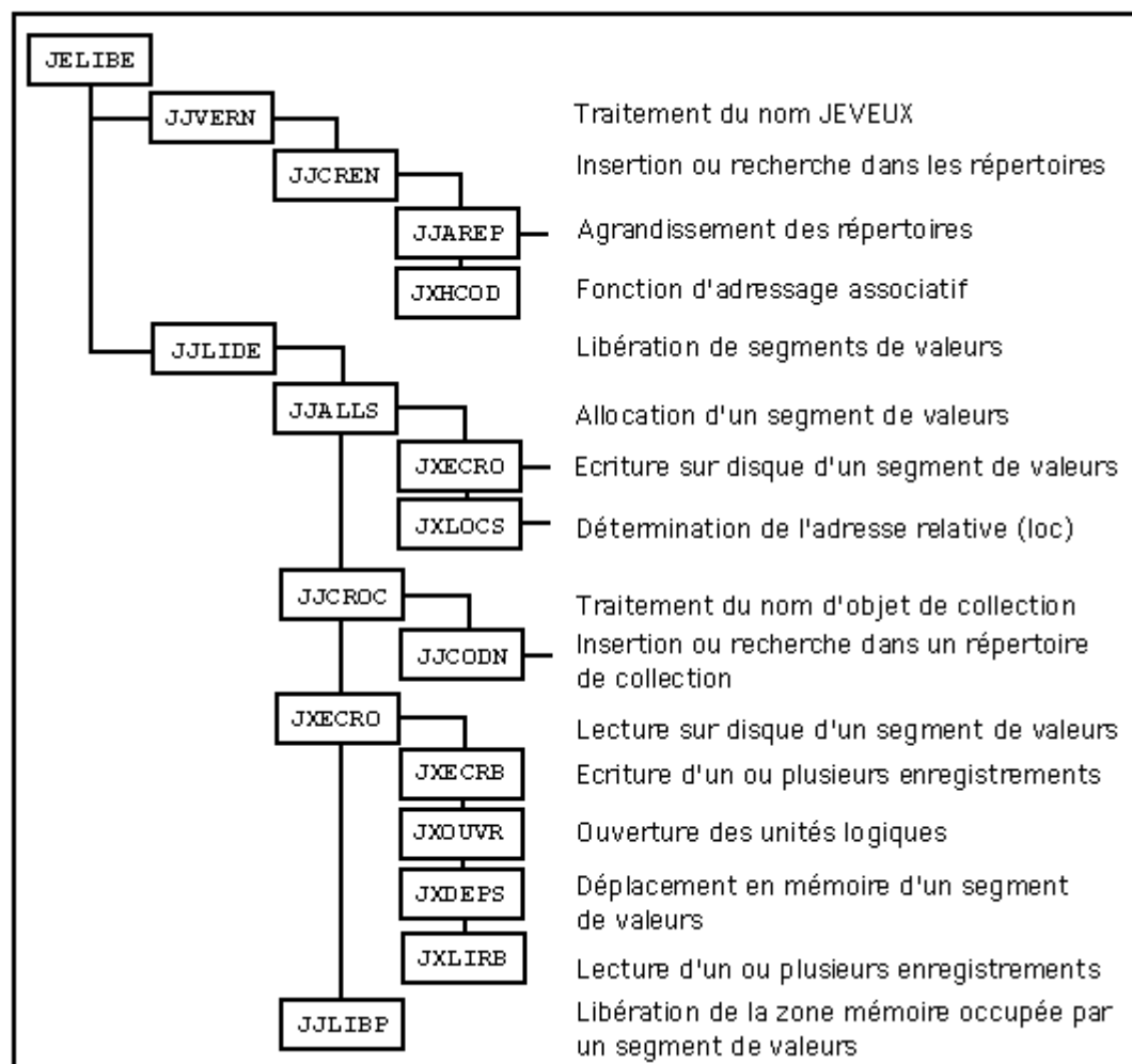
Arbre d'appel de la routine JELIBE
