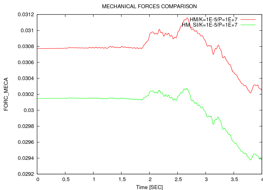
Figure 7.2-d : Comparaison des maxima de forces nœdles mécaniques (estimées) entre les modélisation HM et HM_SI, avec adimensionnement.
