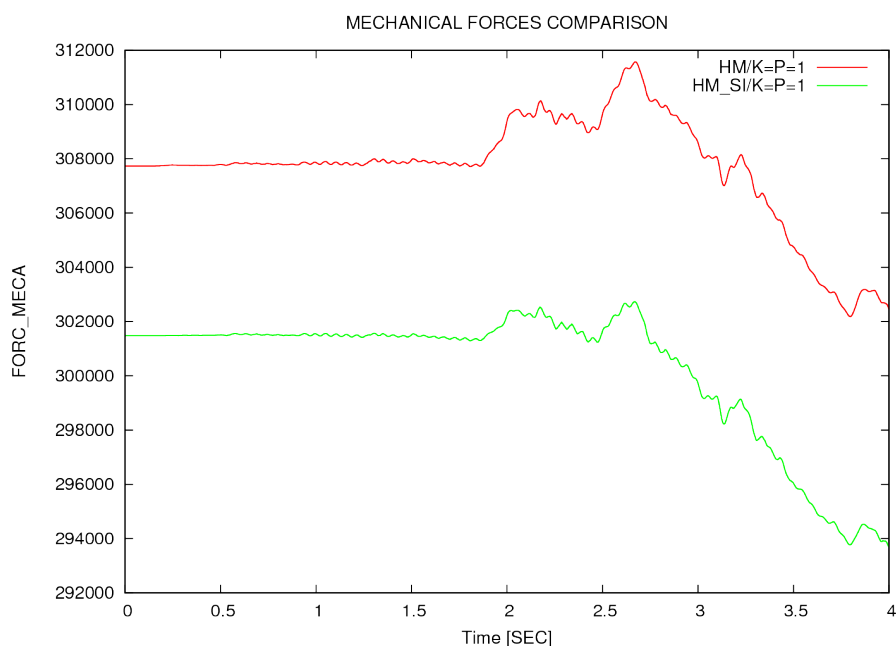
Figure 7.2-c : Comparaison des maxima de forces nodales mécaniques (estimées) entre les modélisation HM et HM_SI, sans adimensionnement.
