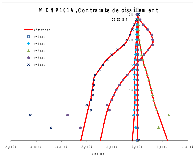
Figure 3.2-b : Répartition de la contrainte de cisaillement le long de la colonne, pour t = 0, 1, 2, 3 et 4 sec. Comparaison avec la solution de référence
