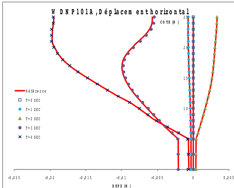
Figure 3.2-a : Répartition du déplacement horizontal le long de la colonne, pour t = 0, 1, 2, 3 et 4 sec. Comparaison avec la solution de référence
