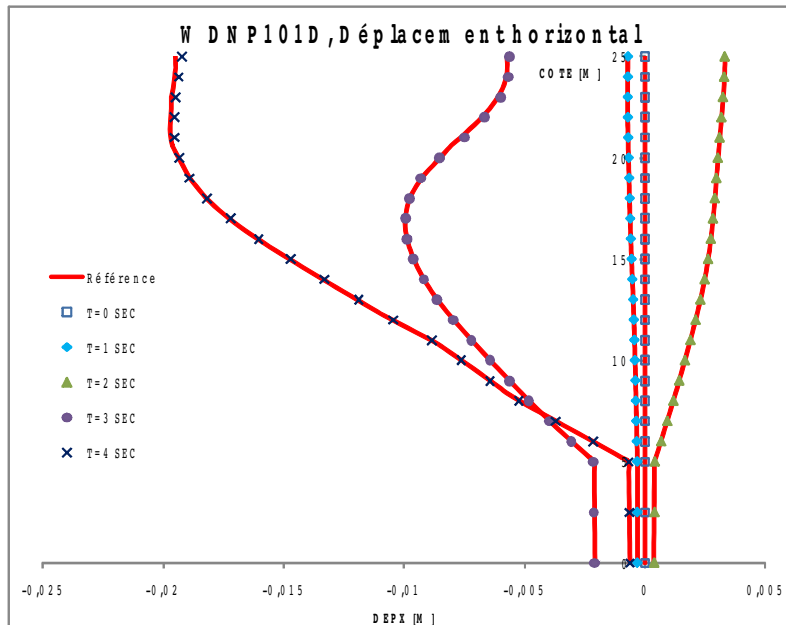
Figure 9.2-a : Répartition du déplacement horizontal le long de la colonne, pour t = 0, 1, 2, 3 et 4 sec. Comparaison avec la solution de référence
