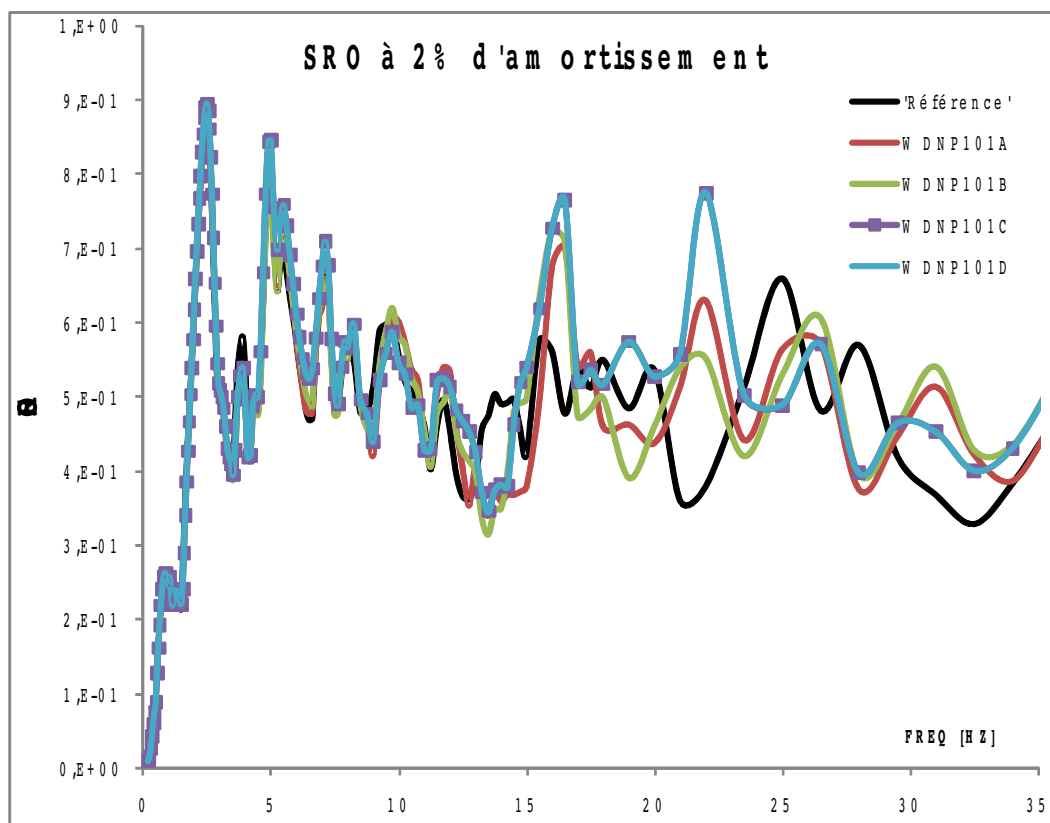
Figure 10-d : SRO au taux d'amortissement de 2% au sommet de la colonne. Comparaison des solutions des modélisations A, B, C et D avec la solution de référence.
