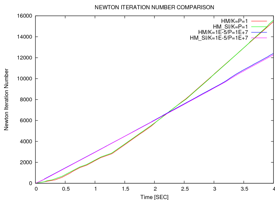
Figure 7.2-b : Comparaison du nombre d'itérations de Newton cumulé entre les modélisations HM et HM_SI, avec et sans adimensionnement.
