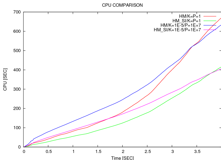
Figure 7.2-a : Comparaison des temps CPU entre les modélisations HM et HM_SI, avec et sans adimensionnement.
