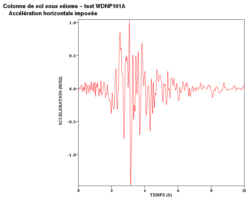
Figure 1.3-a : Accélération horizontale imposée à la base de la colonne.
