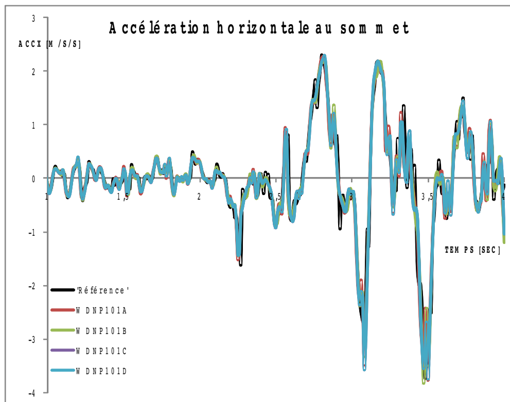
Figure 10-a : Évolution de l'accélération horizontale au sommet de la colonne. Comparaison des solutions des modélisations A, B, C et D avec la solution de référence.
