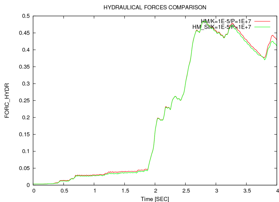
Figure 7.2-f : Comparaison des maxima de forces nodaes hydrauliques (estimées) entre les modélisation HM et HM_SI, avec adimensionnement.
