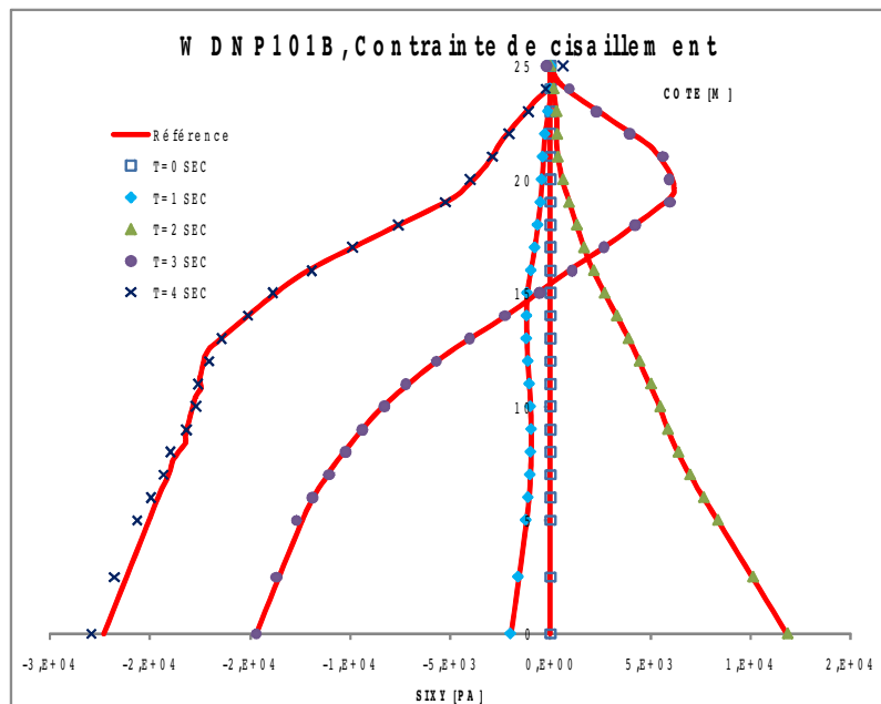
Figure 5.2-b : Répartition de la contrainte de cisaillement le long de la colonne, pour t = 0, 1, 2, 3 et 4 sec. Comparaison avec la solution de référence
