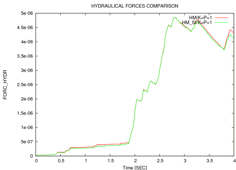
Figure 7.2-e : Comparaison des maxima de forces nœdles hydrauliques (estimées) entre les modélisation HM et HM_SI, sans adimensionnement.
