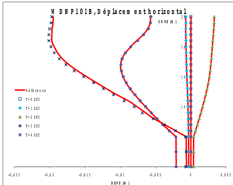
Figure 5.2-a : Répartition du déplacement horizontal le long de la colonne, pour t = 0, 1, 2, 3 et 4 sec. Comparaison avec la solution de référence
