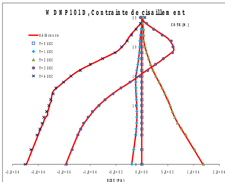
Figure 9.2-b : Répartition de la contrainte de cisaillement le long de la colonne, pour t = 0, 1, 2, 3 et 4 sec. Comparaison avec la solution de référence
