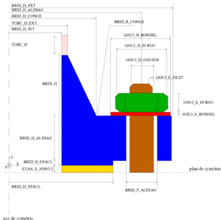
Figure Géométrie de la bride et du goujon.
