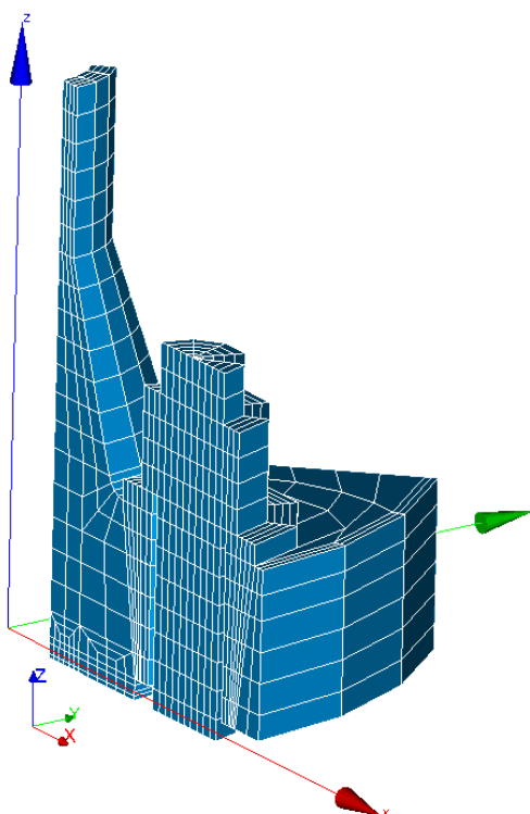
Figure Maillage de la bride et du goujon.
