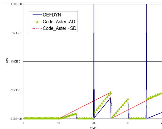
Figure 3-c: rayon déviatoire cyclique en fonction du temps fictif: comparaison entre les solutions de Code_Aster et GEFDYN.
