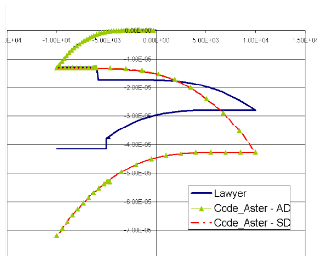
Figure 3-b : déformation volumique plastique cumulée en fonction de la contrainte déviatoire : comparaison entre les solutions de Code_Aster et GEFDYN.
