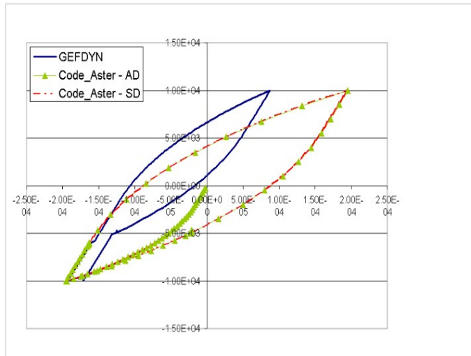
Figure 3-a : Contrainte déviatoire en fonction de la distorsion : comparaison des solutions de Code_Aster et GEFDYN
