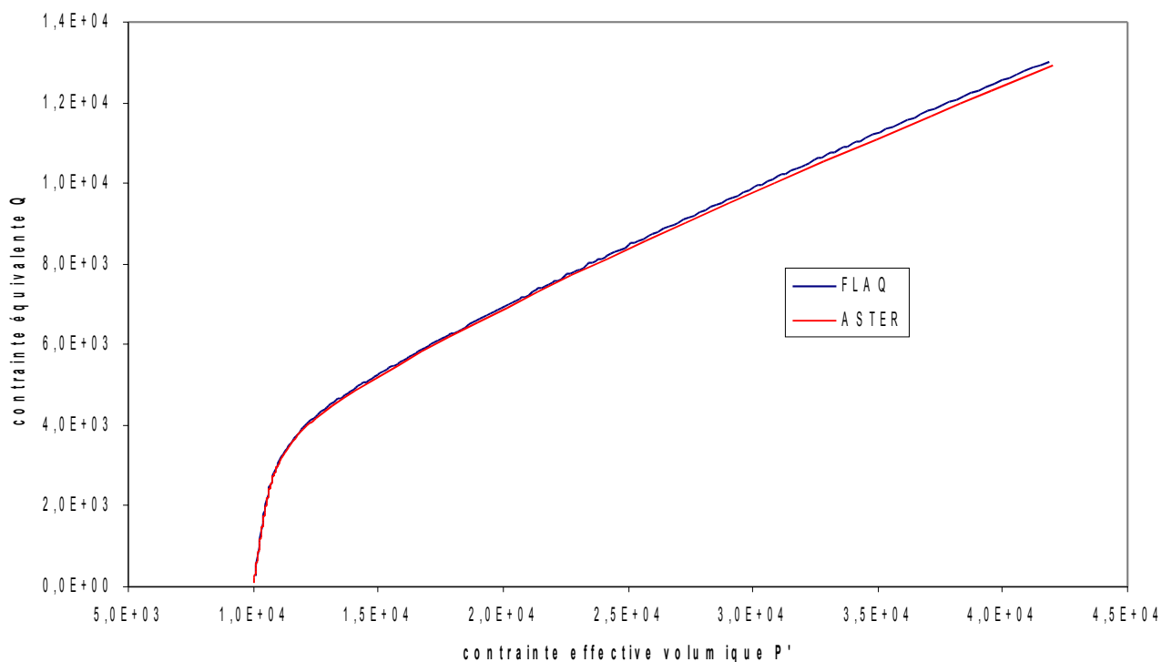
Figure 1 : Trajet de chargement de le plan (P', Q) : comparaison entre les solutions Code_Aster et FLAQ.
