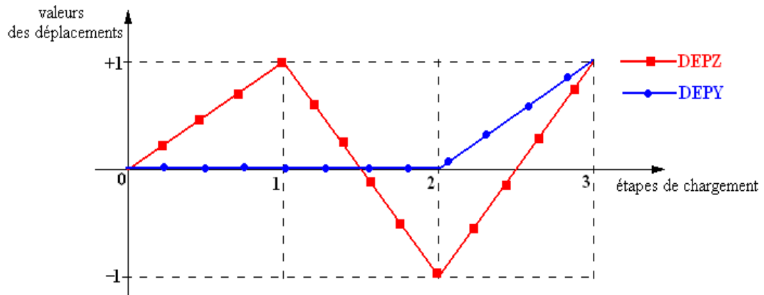
Figure 1.3-1: Variations des chargements en déplacements imposés
