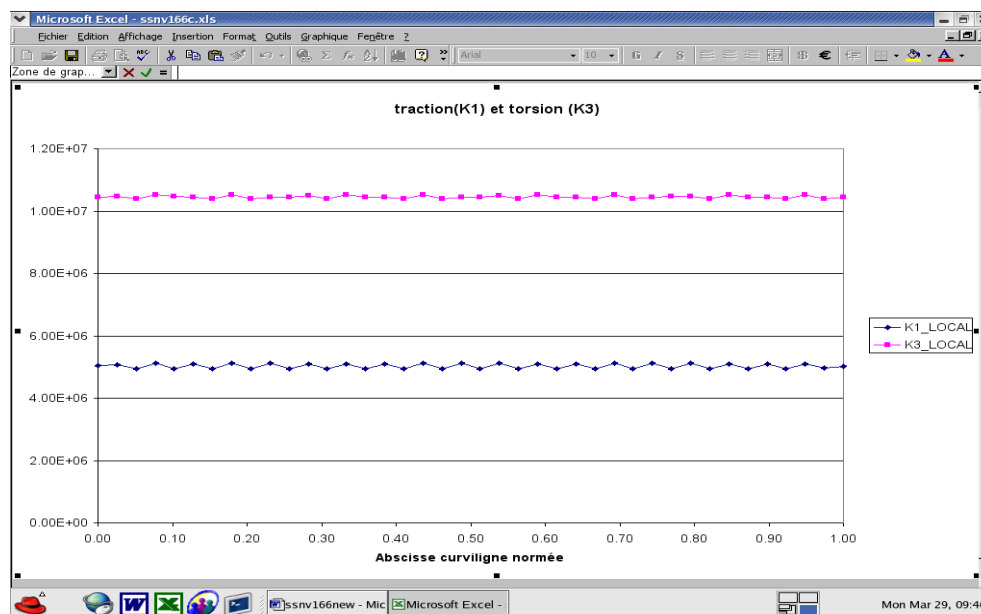
Figure 5.4-a : K1 et K3 le long du fond de fissure (en MPa.m^{1/2} )
