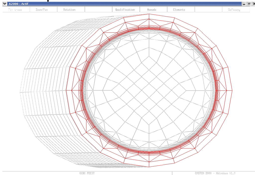
Figure 3.1 - a : Coupe du maillage dans le plan de la fissure
