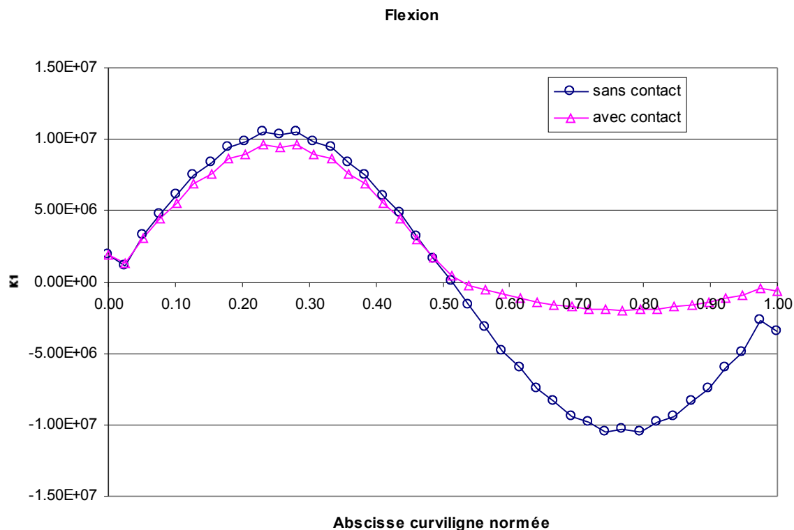
Figure 5.4-b : K_I le long de la fissure (en \text{MPa.m}^{1/2} )
