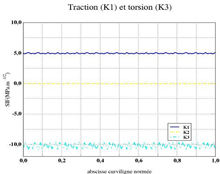
Figure 4.4-a : K1 , K2 et K3 le long du fond de fissure (en \text{MPa}\cdot\text{m}^{1/2} )
