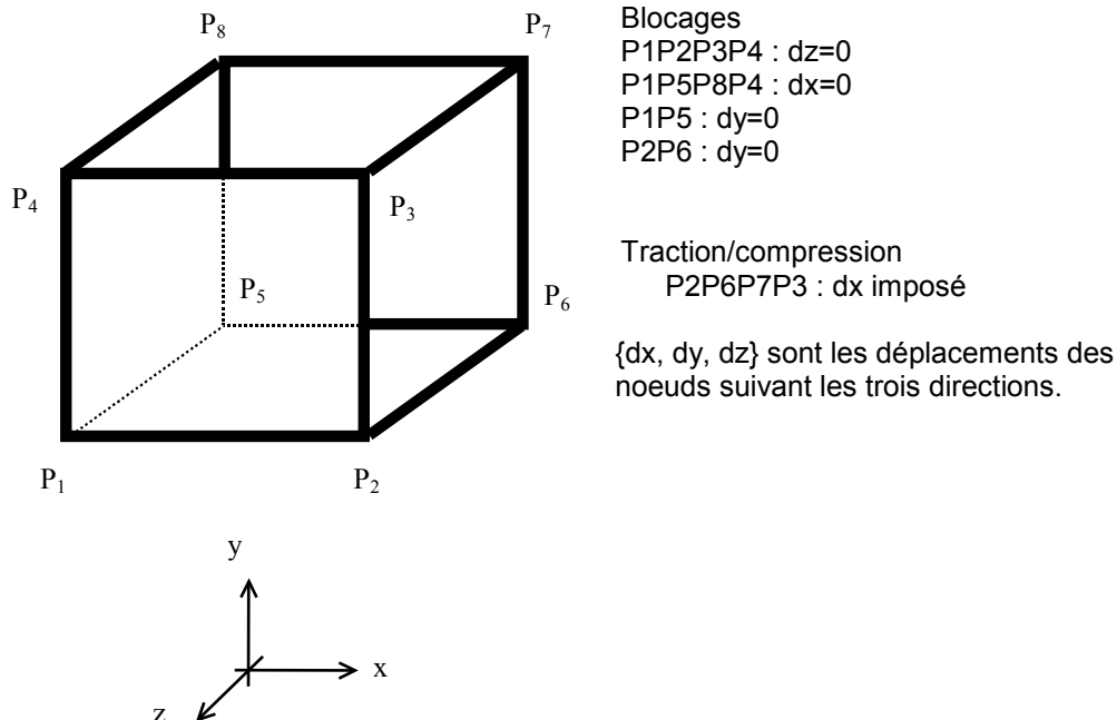
Figure 1.1-a : Géométrie et conditions aux limites des tests uniaxiaux
