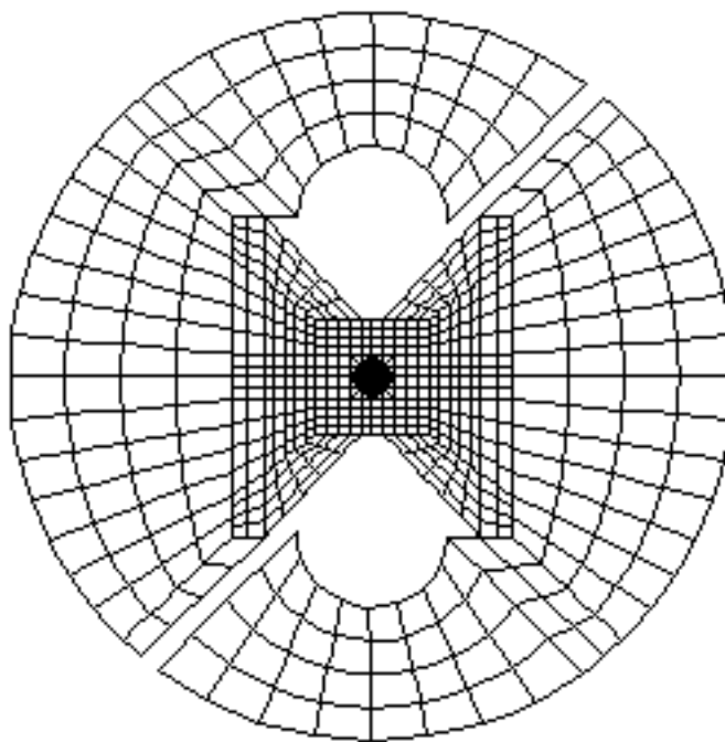
Maillage de l'éprouvette et du porte éprouvette
