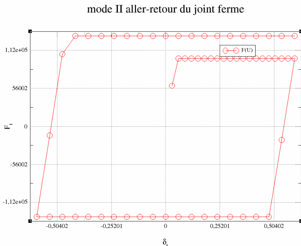
Illustration 2: Courbe force (tangente) déplacement pour la loi JOINT_MECA_FROT
