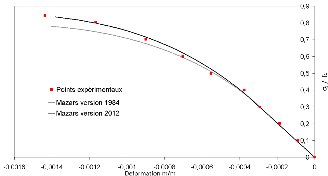
Figure 2.1-b : Comparaison des courbes expérimentale et numériques lors de l'essai biaxial \omega = 0.52
