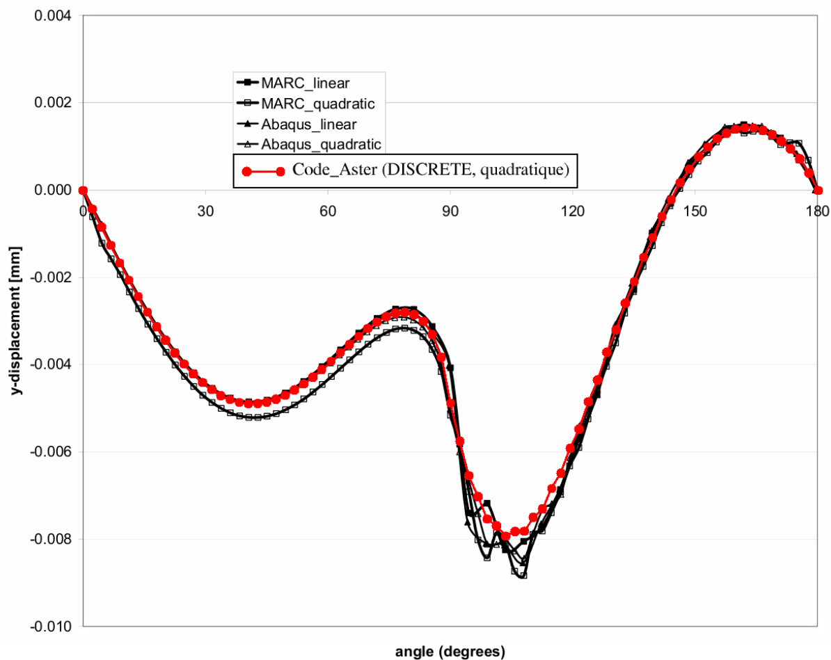
Illustration 4: comparaison entre MARC, Abaqus et Code_Aster (déplacement suivant y du poinçon)
