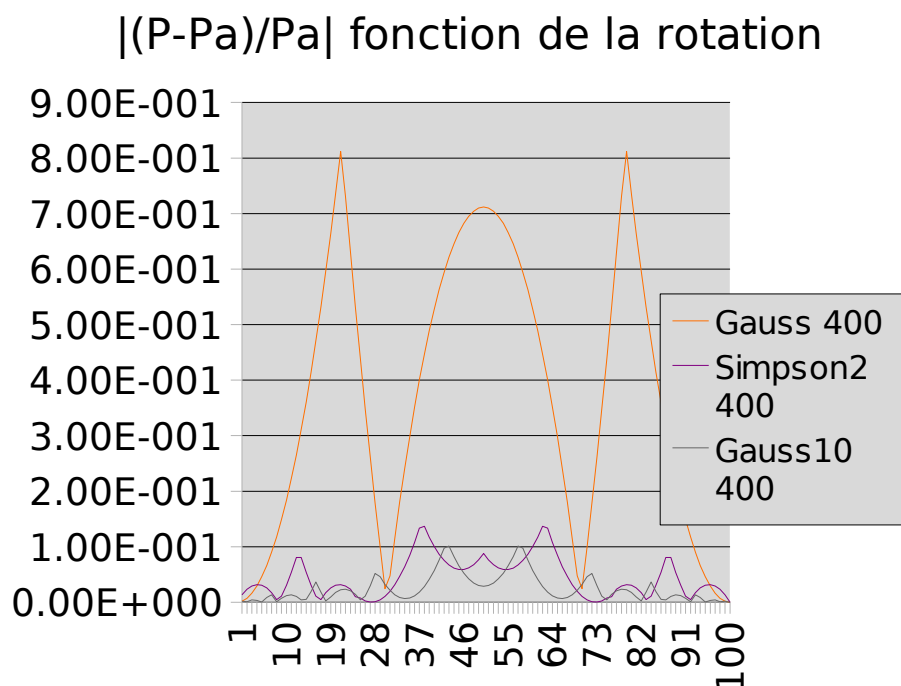
Figure 5.4-3: Evolution de la pression de contact lors de la rotation pour 1600 éléments sur la circonférence R=R_2 pour une couronne intérieure rigide. Une intégration avec 2 points de Gauss conduit à une erreur maximale de 80%. Seules les intégrations de Gauss à 10 et de Simpson à l'ordre 4 permettent de ramener l'erreur maximale aux alentours de 15% pour des maillages incompatibles.
