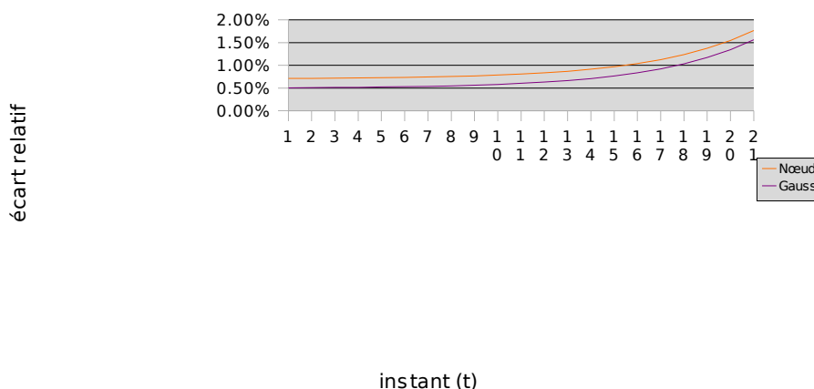
Figure 4.4-1: évolution de l'écart entre la solution analytique et la solution donnée par Code_Aster pour une intégration aux nœuds et aux points de Gauss.
