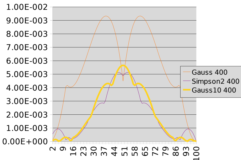
Figure 9.3-2: Evolution de la pression de contact lors de la rotation pour 1600 éléments sur la circonférence R=R_2 pour un disque intérieur rigide. L'ensemble des schémas de Gauss à l'ordre 3, Gauss à l'ordre 10 et Simpson à l'ordre 4 donne une erreur inférieure à 1%. Un schéma au nœud donne une erreur constante sur l'ensemble de la rotation de 33,4% non représentée ici.
