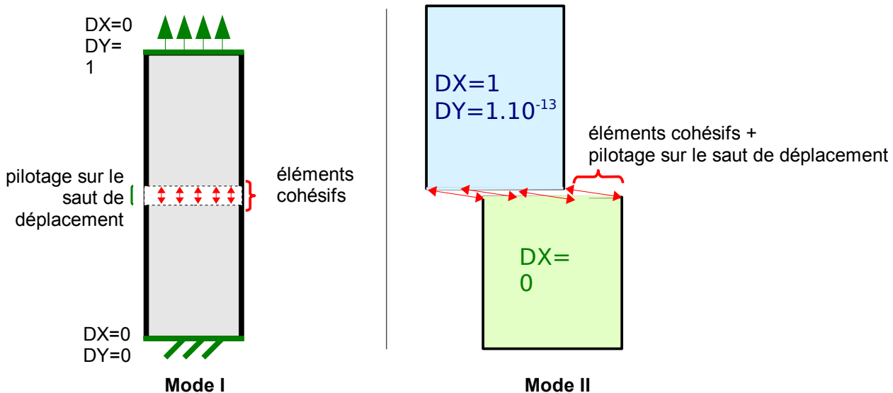
Figure 1.4.2-1: Chargement appliqué, en mode I et en mode II
