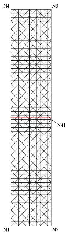
Figure 6.2-a: Maillage de la modélisation D
