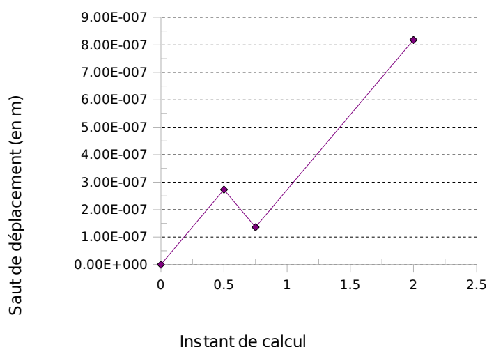
Figure 1.5-1: Évolution du saut de déplacement imposé par pilotage jusqu'à l'instant de calcul 2.
