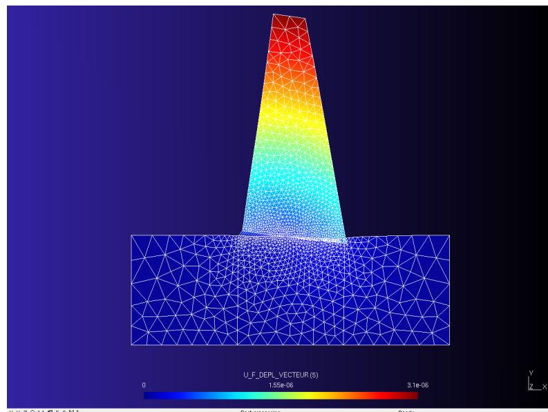
Figure 3.3 : Déformée du barrage et ouverture de la fissure
