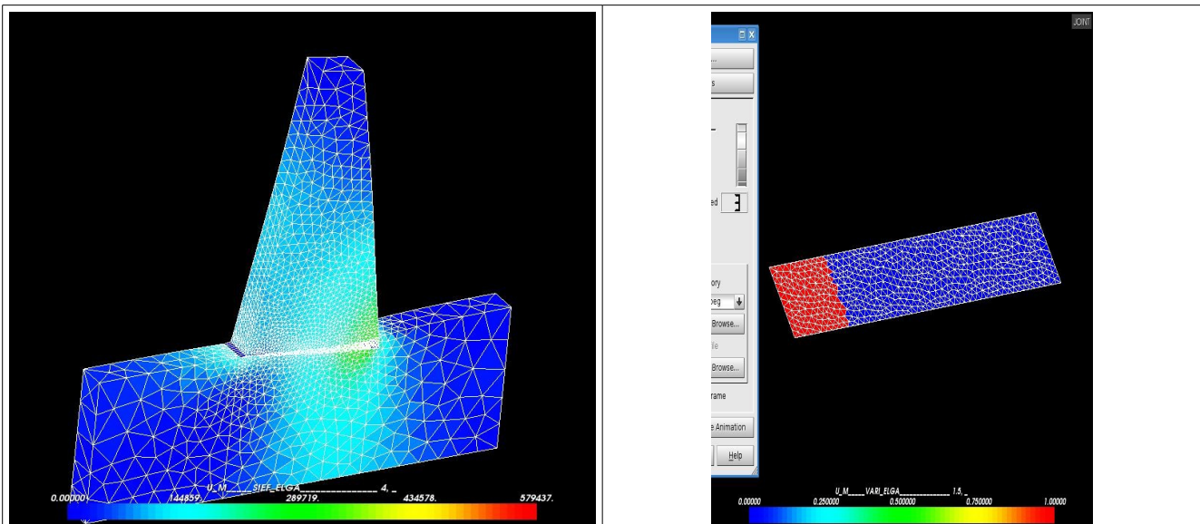
Figure 6.3 : Contraintes sur le barrage et la partie du joint en glissement (en rouge)
