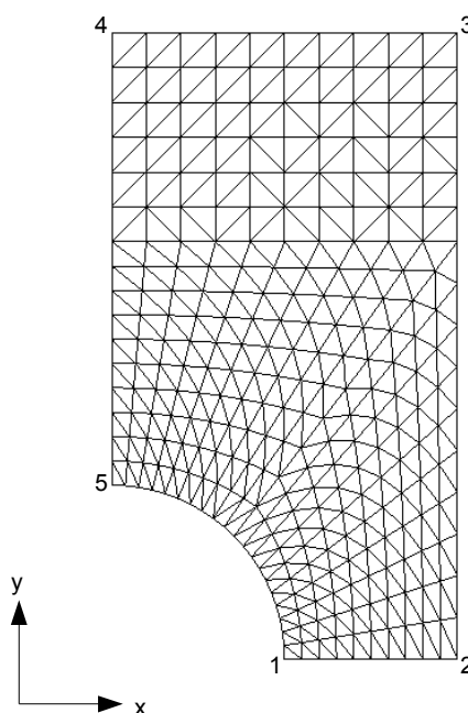
Figure 3.1-a: Maillage de la modélisation A
