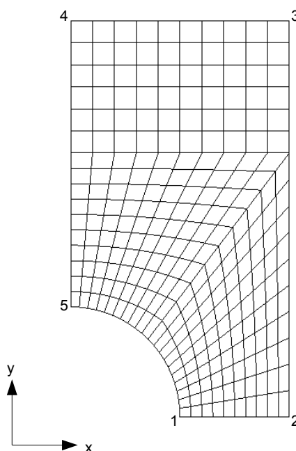
Figure 4.1-a: Maillage de la modélisation B
