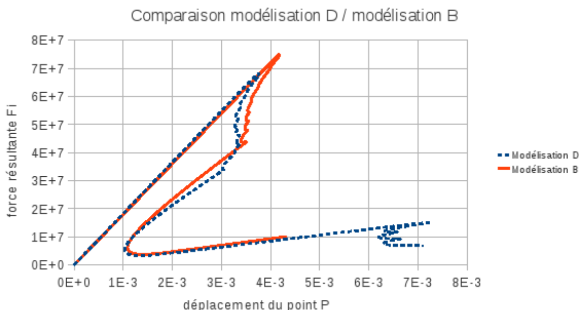
Figure 6.3-a: comparaison éléments de joint avec éléments à discontinuité interne.
