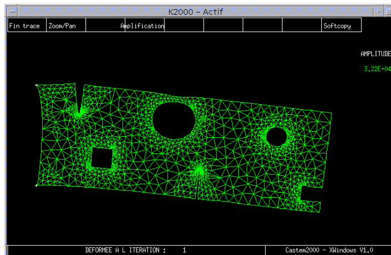
Figure 1.1-e : Déformée du maillage mécanique (modélisation B)
