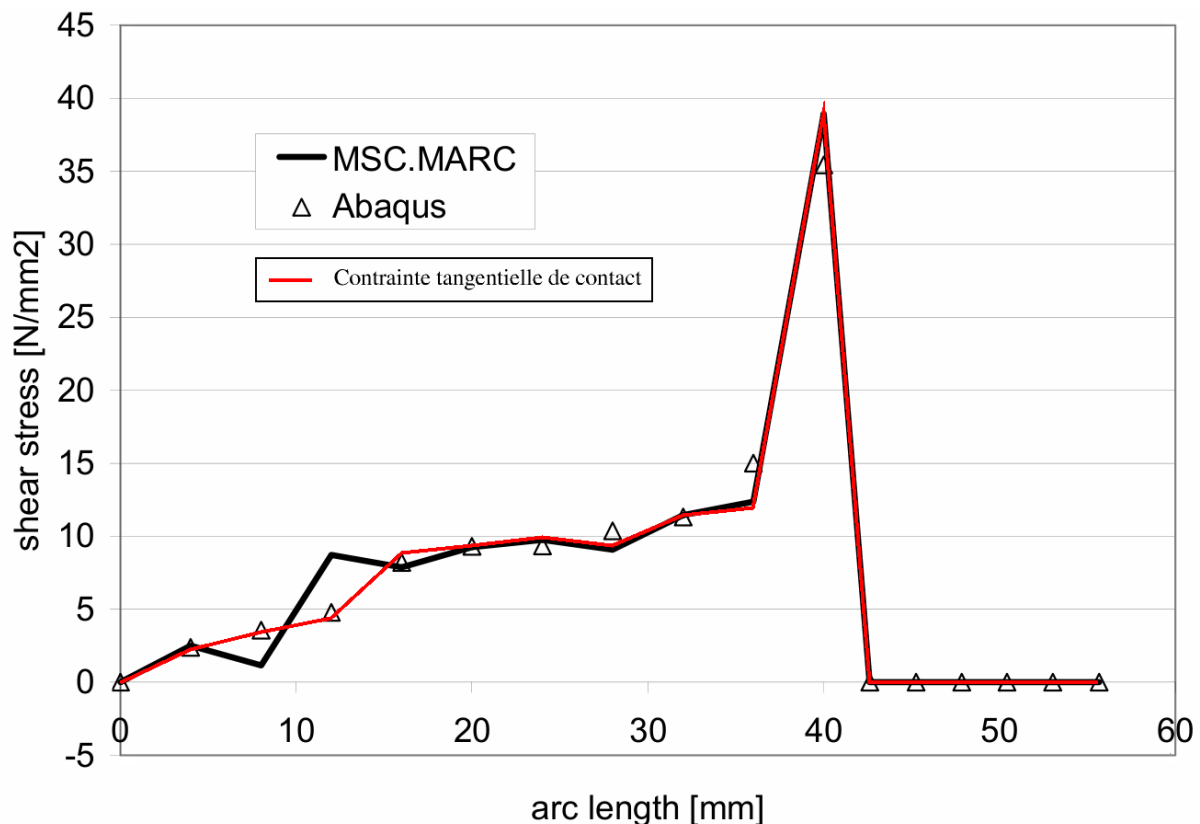
Illustration 1: Comparaison de la contrainte tangentielle entre Abaqus, MARC et Code_Aster
