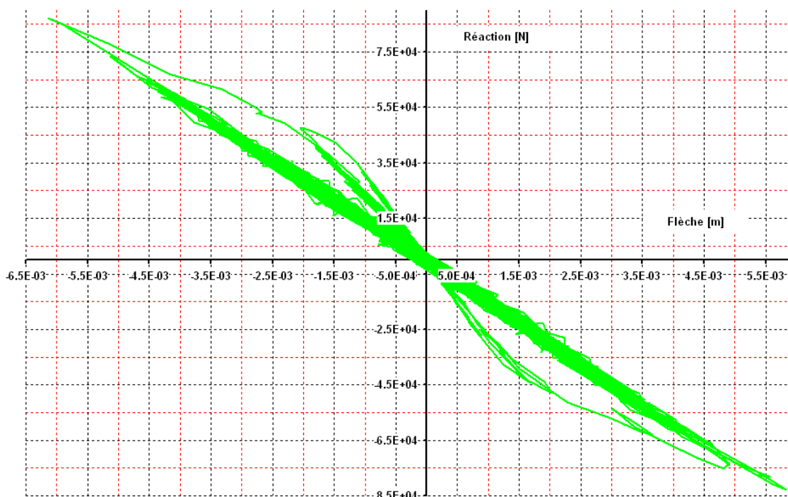
Figure 4.2-f: Courbe réaction-flèche, pour 15 secondes.
