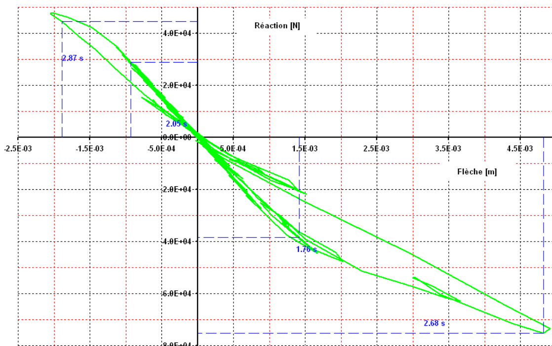
Figure 4.2-c : Courbe réaction-flèche pour les 3 premières secondes.
