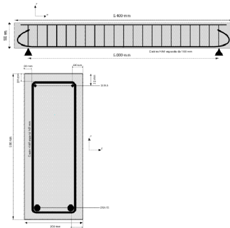
Figure Géométrie de la structure
