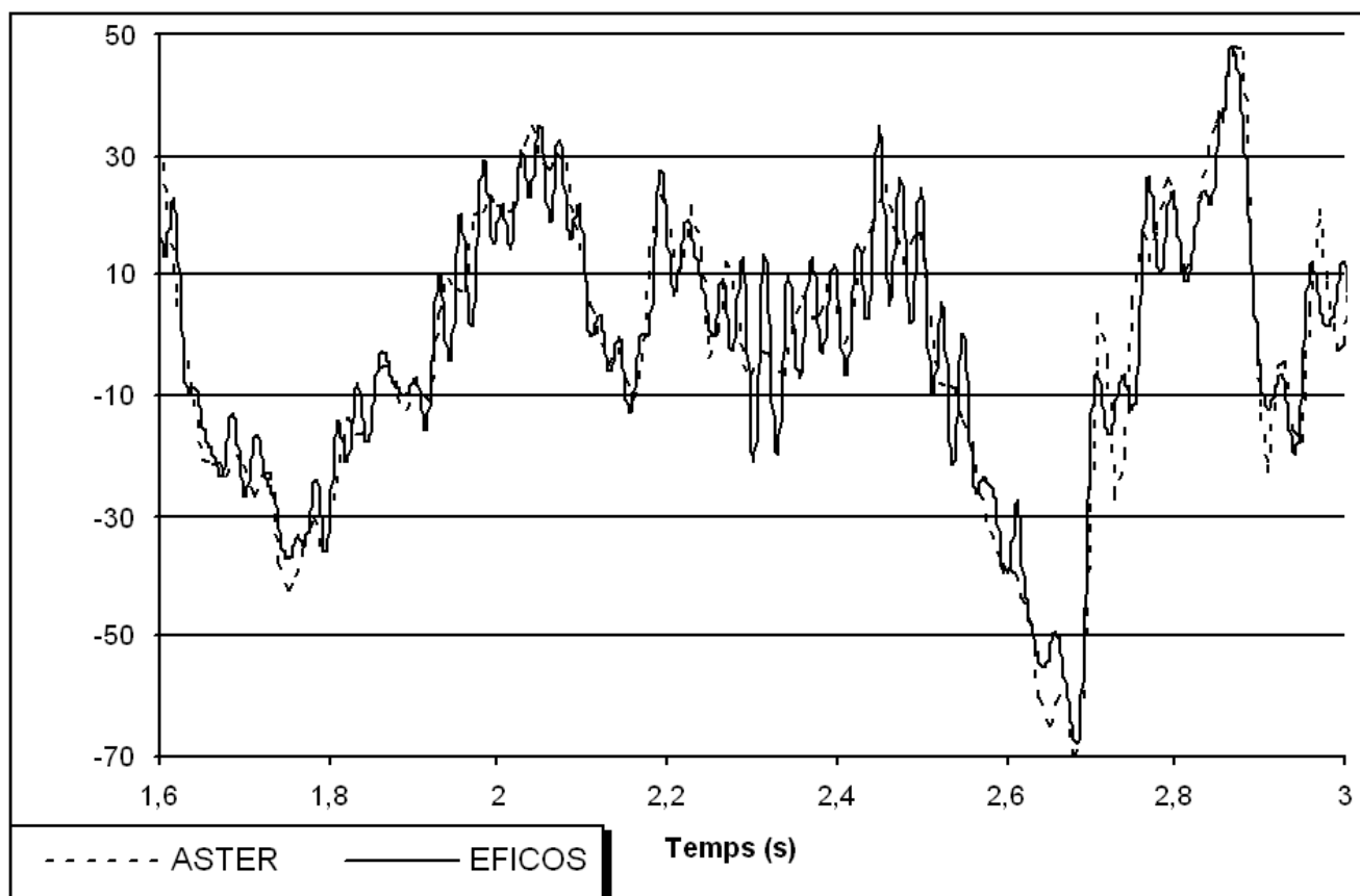
Figure 3.2-b : Détail de la réaction entre 1,6 et 3 secondes
