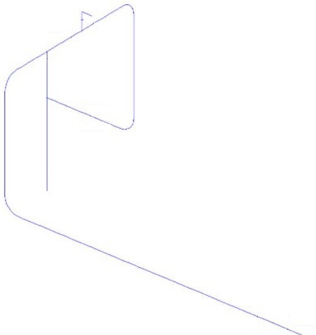
Figure 3.1-a : Maillage.
