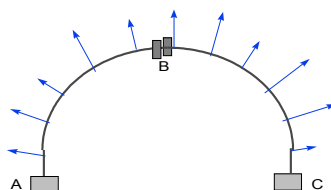
Figure 1.1-a : Schéma de la zone cintrée d'un tube de GV, supposé être encastré en dernière plaque entretoise, guidé dans un support à jeu
