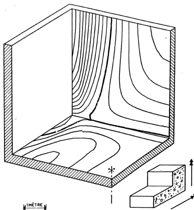
Fig. 14. — Cuve carrée en béton armé. Tracé des iso-moments M_{xx} (pas : 10^6 Nm par mètre).
