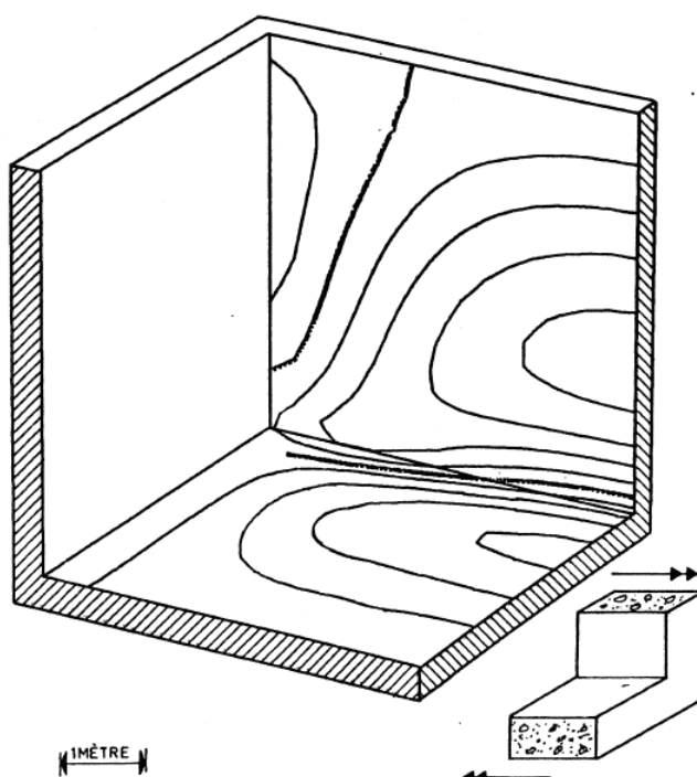
Fig. 15. — Cuve carrée en béton armé. Tracé des iso-moments M_{yy} (pas : 10^6 Nm par mètre).
