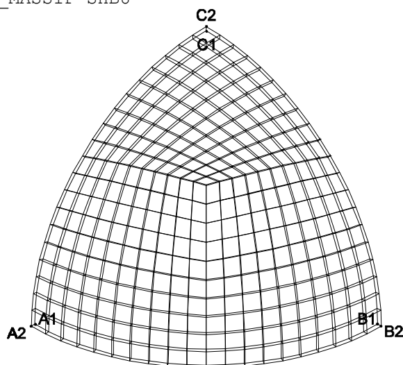
Modélisation d'un quart de l'hémisphère en SHB8
