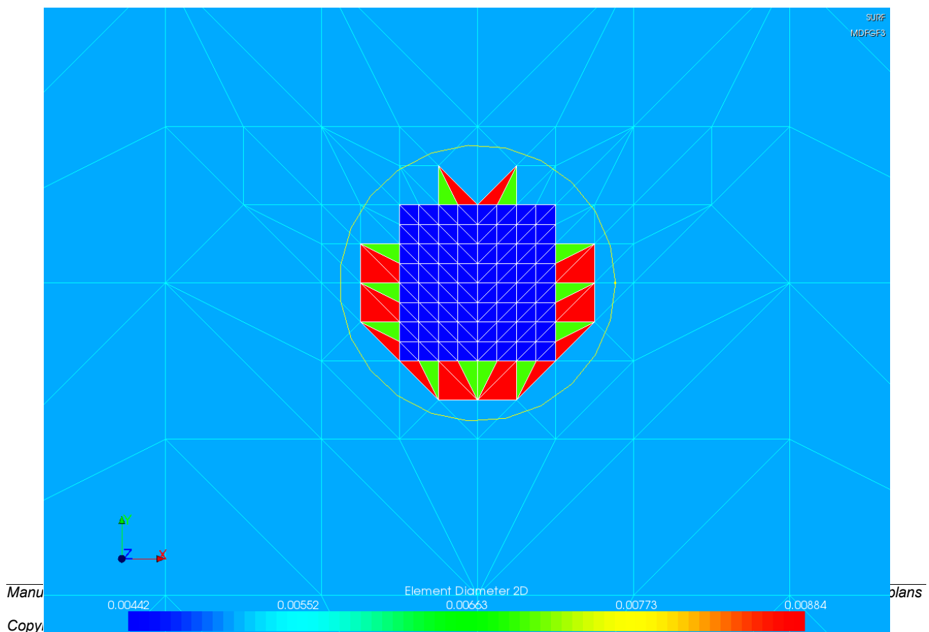
Figure 4.2-3: maillage sain raffiné - zoom autour du fond de fissure n°1 de la fissure centrée en A et carte de tailles dans la zone d'intérêt
