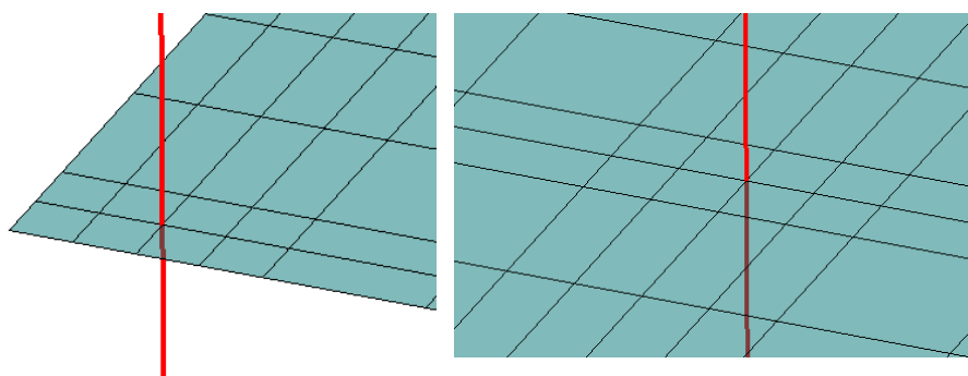
Figure 5-b : Détail du maillage autour des poteaux de rive et central.
