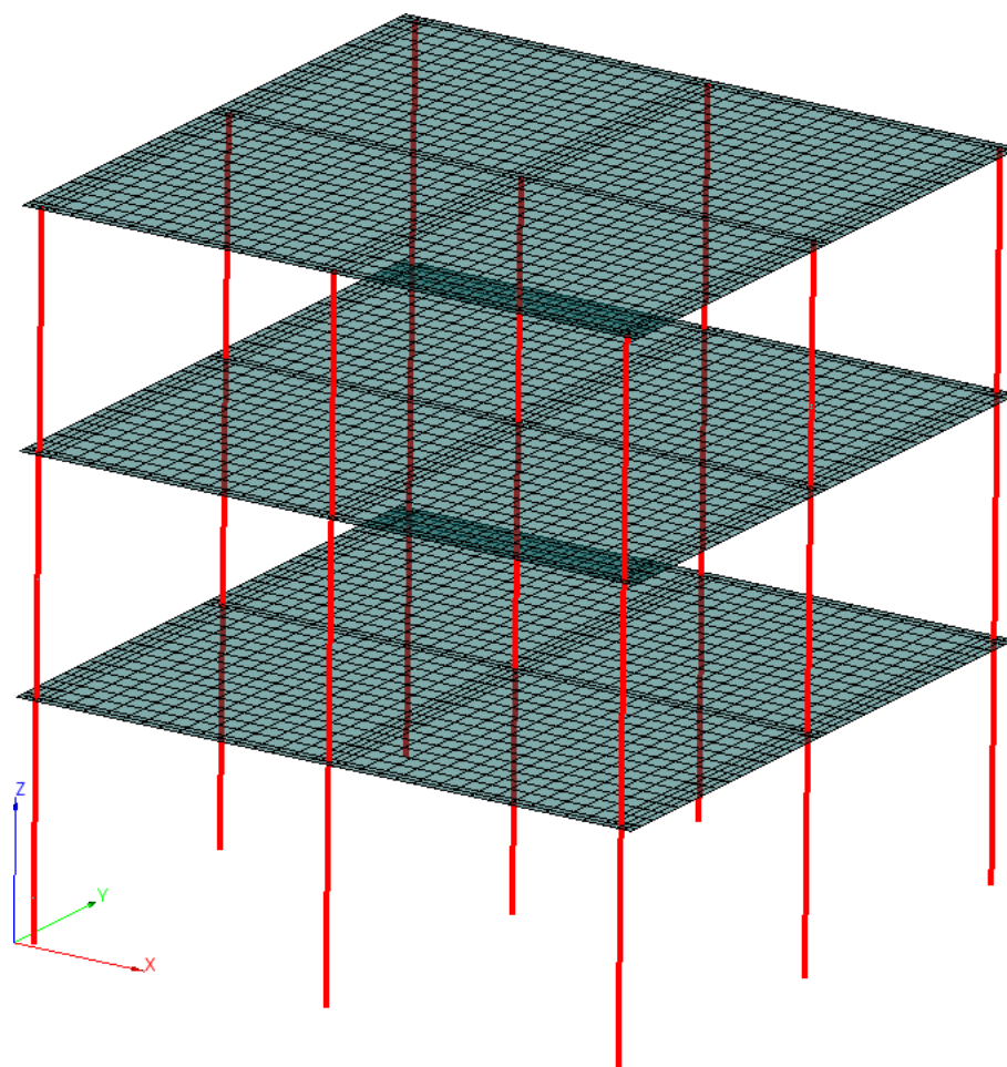
Figure 5-a : Maillage du bâtiment.
