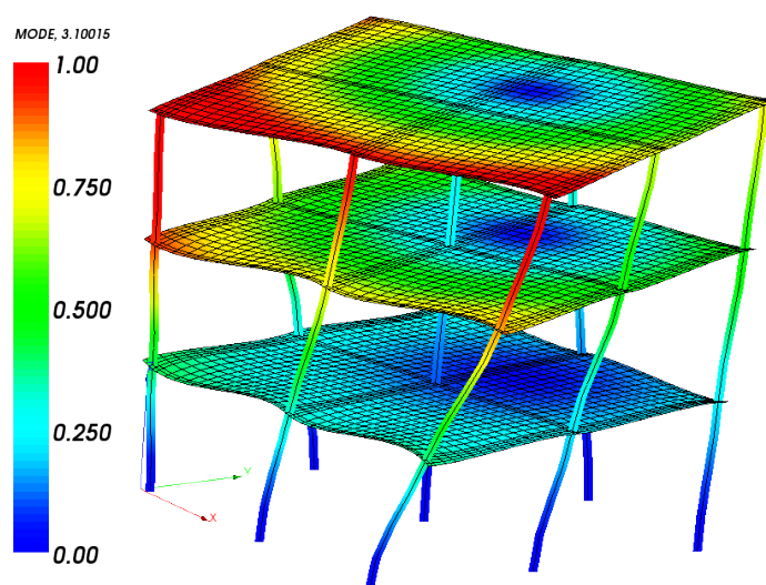
Figure 5-c : 3 ème mode propre, modélisation B.
