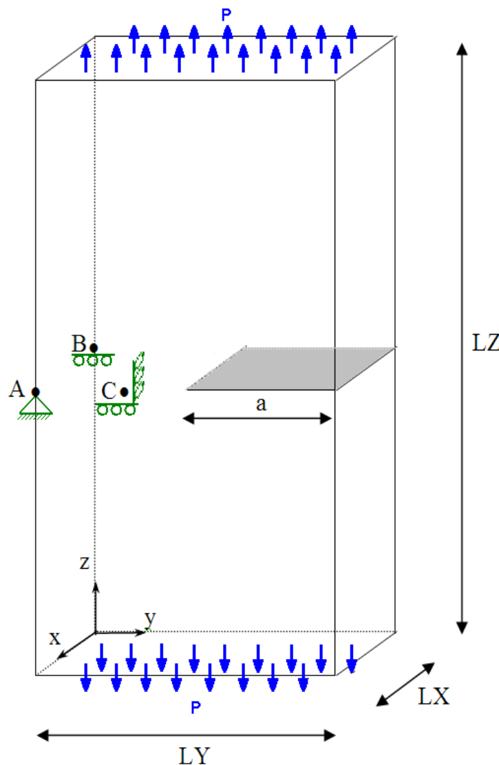
Figure 1.1-1.1-a : Géométrie de la plaque fissurée avec illustration du chargement et des conditions aux limites
