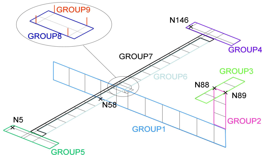
Figure 1-1: maillage du modèle numérique
